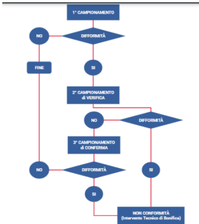
Figura 3 - Flusso di verifica conformità analisi qualitative dei gas
